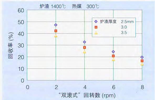
图4 “双滚式”间接冷却的热回收装置计算结果
