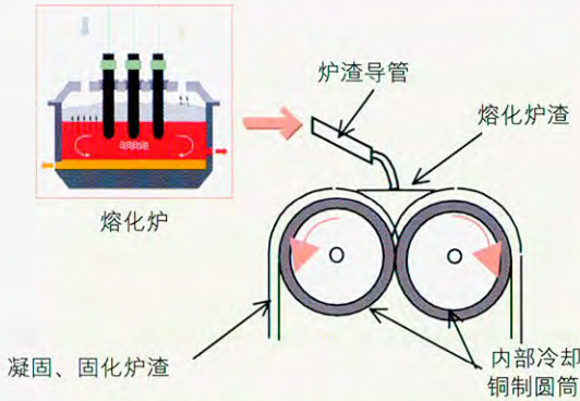
图1 “双滚式”炉渣间接冷却装置
