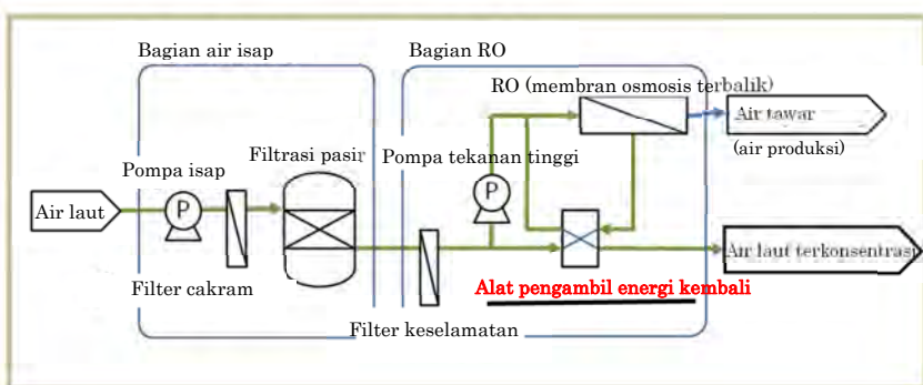
Alur Desalinasi air laut
